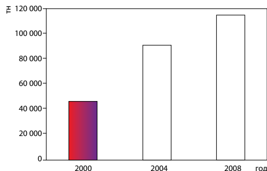
Рис.1. Динамика объемов потребления безгалогенных композиций в европейской кабельной промышленности
